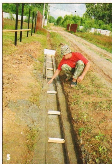
5 Ширины фанерных полос не хватало для формирования полноценного арочного свода, поэтому стенки трубы «подняли», залив пару полосок бетона.
