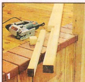
Стойки и стропила перголы выкраивают из досок сечением 45х95 мм. Для крепления к цоколю террасы в стойках на соответствующем расстоянии от нижнего торца выбирают пазы.
