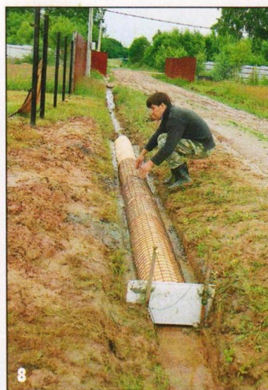
8 При установке арматуры свода надо было обеспечить зазор между сеткой и фанерной опалубкой.
