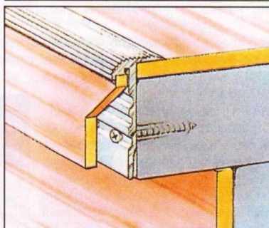
Рис. 2. Если проступь ступени выступает вперёд — в профиль под нижнюю губку вклеивается фасадный щиток из ламината.
