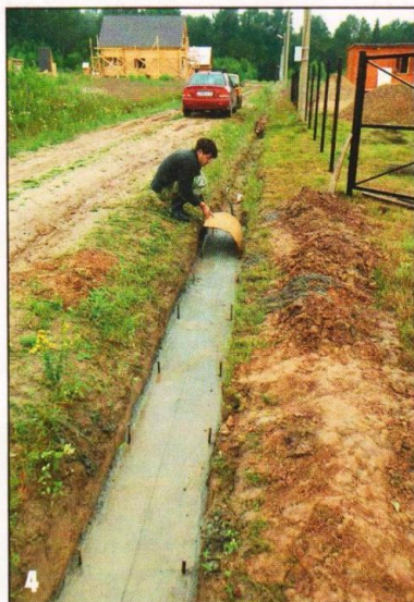
4 При заливке бетона замонолитили отрезки арматуры, чтобы связать основание трубы с будущим сводом (фото 4). Кстати, ряд этих штырей помог нам выбрать типоразмер листов фанеры, которых в наличии было немного и поэтому хотелось их использовать оптимальным образом. Ширины листа, который
