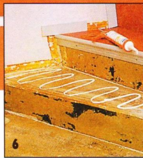
6 Выкроенные элементы облицовки крепят к ступеням на монтажном клее, который обильно наносят змейкой на проступь.
