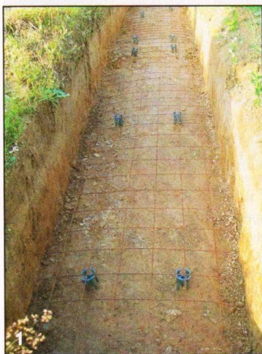
Арматурную сетку в отрытую траншею устанавливали на пластиковые «стульчики», чтобы при заливке бетона сетка не упала на землю.
